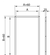
RAMKA PODTYNKOWA RWX
