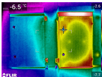
Rys. 1 Z lewej strony widoczna obudowa Galvar z zamontowaną termoizolacją typu Premium 20 mm, z prawej strony analogiczna obudowa, ale bez termoizolacji. W obudowy obudowach włączone jest źródło ciepła w postaci grzałki o mocy 150W. Wyraźnie widać różnicę pokazującą większe straty ciepła przez obudowę bez termoizolacji.
