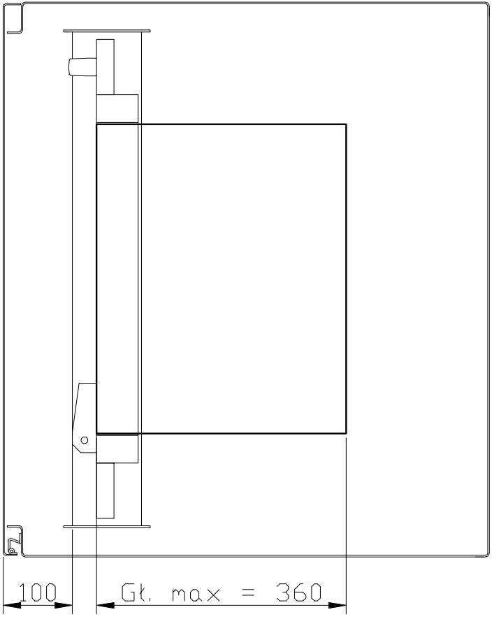
RAMA UCHYLNA SYMETRYCZNA
